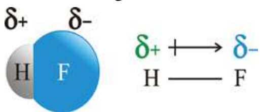
الشكل (2): تمثيل الرابطة القطبية في جزيء \text{H-F}
