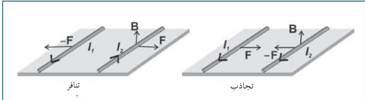
الشكل (7-9): اتجاه القوة المغناطيسية بين سلكين طويلين.
