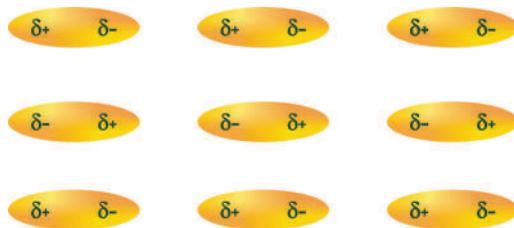
شكل (6): ترتيب الجزيئات القطبية لمركَّب في الحالة السائلة الشكل (6:ب): ترتيب الجزيئات القطبية لمركَّب في الحالة الصلبة
