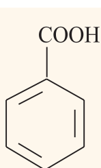
حمض البنزويك
