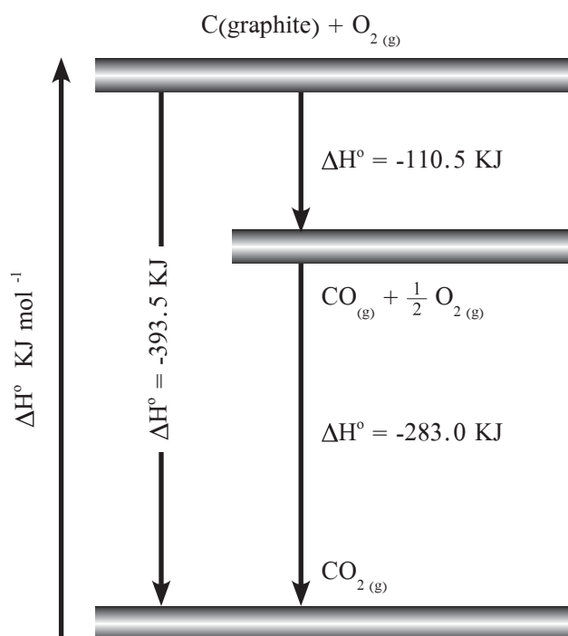
الشكل (7): حساب المحتوى الحراري لـ \text{CO}_2 بشكل غير مباشر
