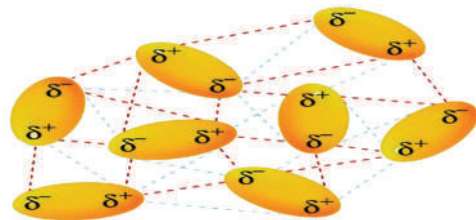
شكل (6): ترتيب الجزيئات القطبية لمركَّب في الحالة السائلة الشكل (6:ب): ترتيب الجزيئات القطبية لمركَّب في الحالة الصلبة
