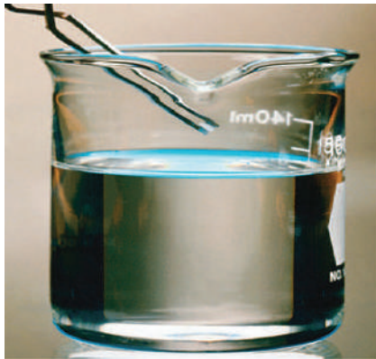
الشكل (3): تبلور أسياتات الصوديوم من محلوله فوق المشبع
