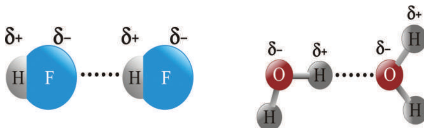
الشكل (7): تمثيل الترابط الهيدروجيني بين جزيئات H 2 O، والترابط الهيدروجيني بين جزيئات HF
