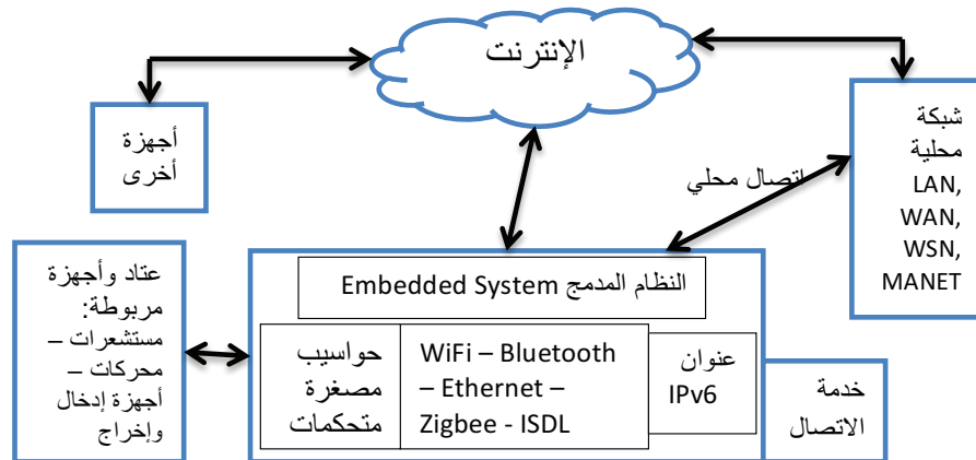
هيكلية مبسطة لنظام إنترنت الأشياء (IoT)
