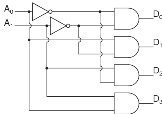
الدارة المنطقية للتركيب الداخلي لوحدة فك شفرة (2-4 decoder)
