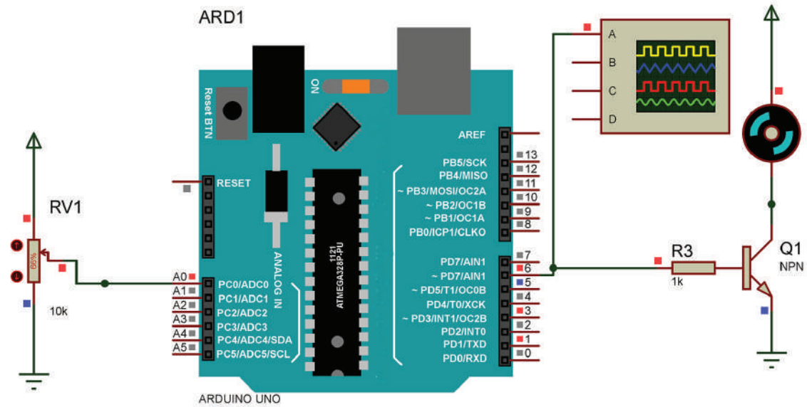
مخطط دارة التحكم بسرعة محرك تيار مستمر باستخدام تقنية PWM
