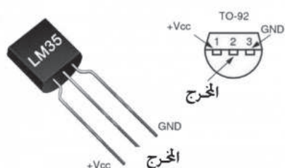
LM35 مستشعر الحرارة
