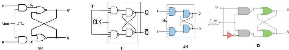
أنواع النطاطات وتركيبها الداخلي
