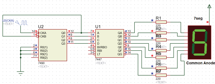
(دارة عدّاد بمنزلة عشرية واحدة)
