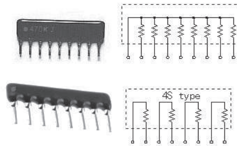
المقاومات الشبكية في النظام التماثلي
