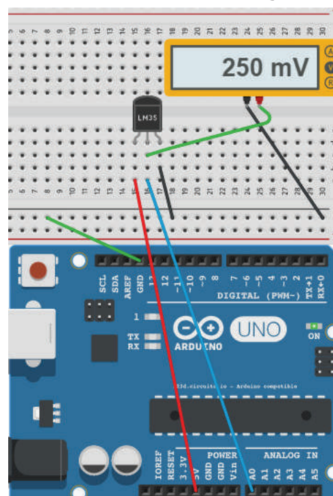
توصيل مستشعر الحرارة مع لوحة الأردوينو
