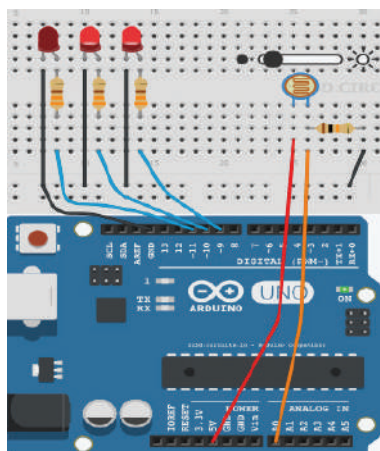
توصيل دائرة مقياس شدة الإضاءة
