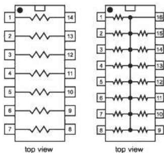
المقاومات الشبكية السطحية
