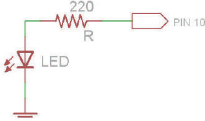
توصيل ثنائي ضوئي بلوحة الأردوينو
