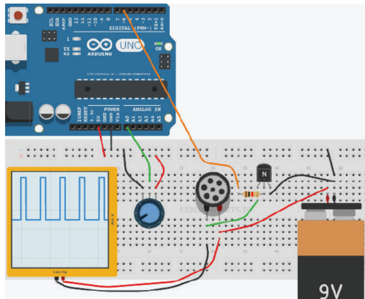
التوصيل العمليّ للدارة في نشاط 4
