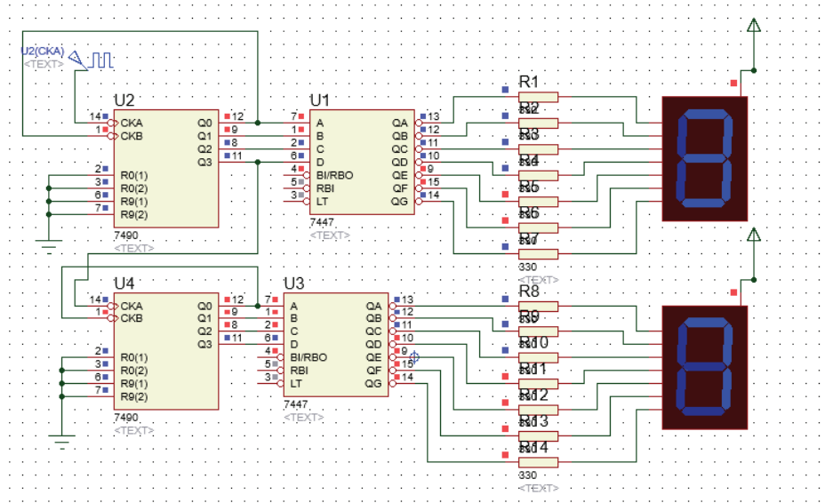
(دارة عدّاد بمنزلة عشرين عشرين)
