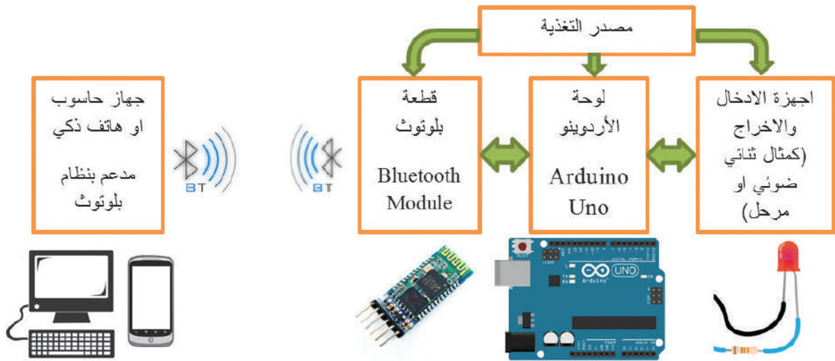
المخطط الصندوقي لنظام تحكم عن بعد عبر اتصال بلوتوث
