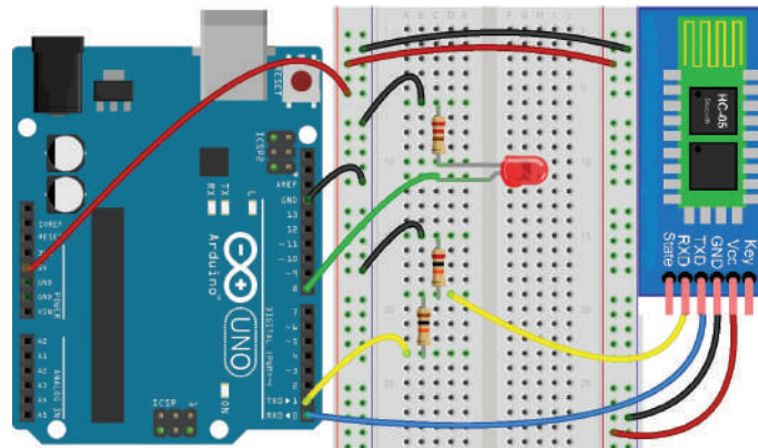
توصيل وحدة البلوتوث مع الأردوينو
