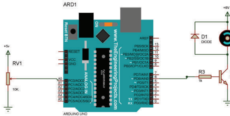
مخطط دائرة التحكم بسرعة محرك تيار مستمر باستخدام تقنية PWM
