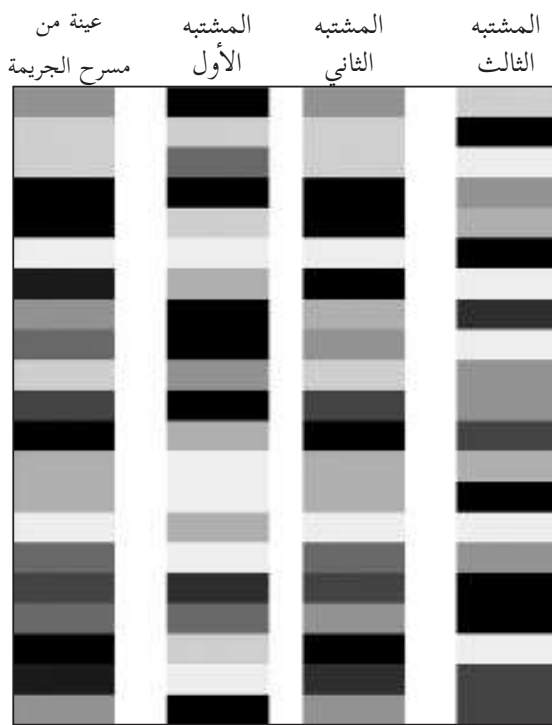
الشكل (٣-٦) تتابعات البصمة الوراثية لثلاثة مشتبهين بجريمة
