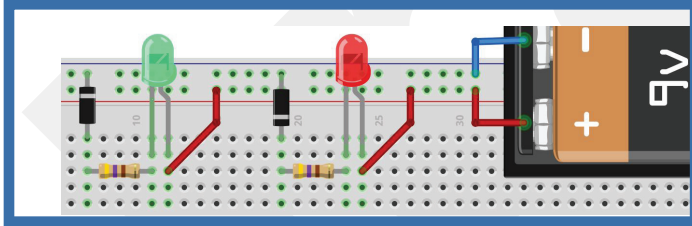
مخطط فحص الثنائي
