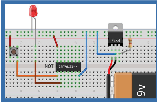
دارة البوابة NOT
