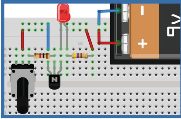
مخطط الدارة التماثلية
