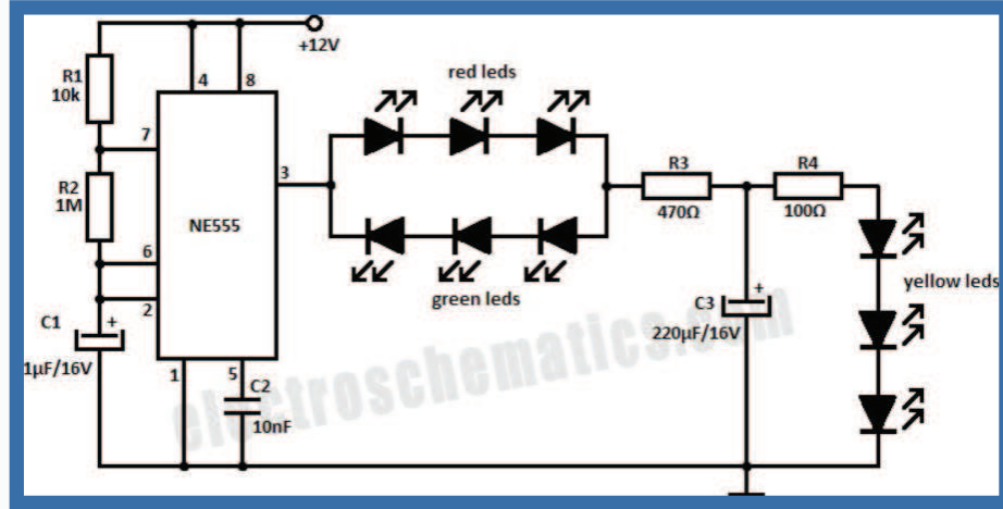
دائرة إشارة المرور باستخدام دائرة المؤقت 555 و المكثفات.
