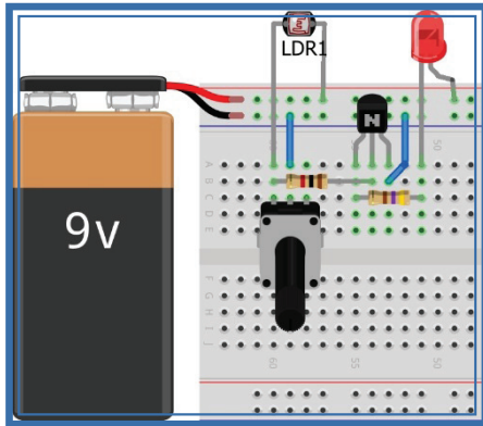
دائرة تحديد الوقت
