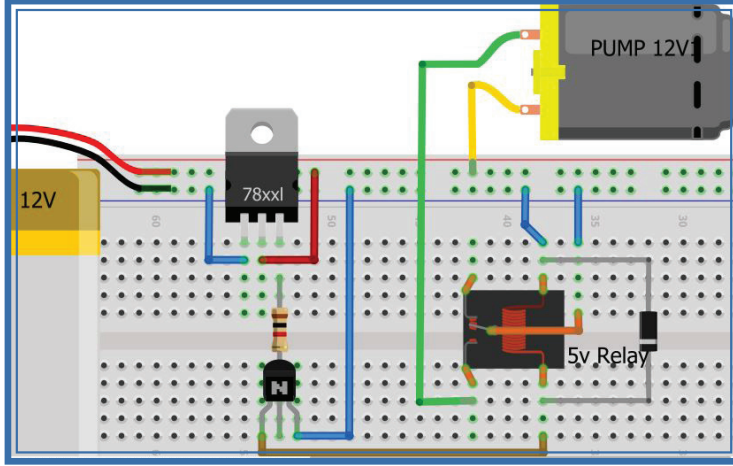
دارة المضخة
