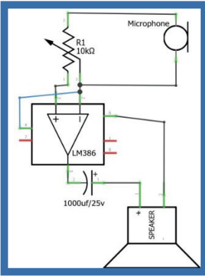
مخطط دارة الصوت
