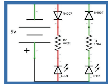
دارة فحص الثنائي
