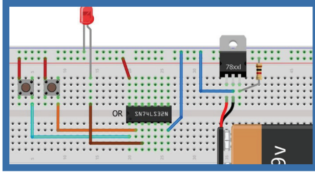
دائرة البوابة OR
