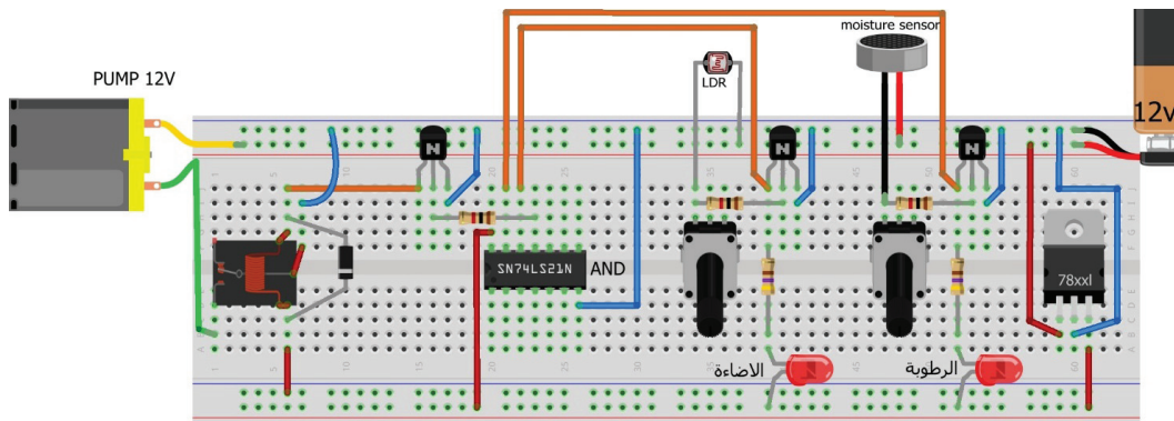
دائرة الري الأوتوماتيكي
