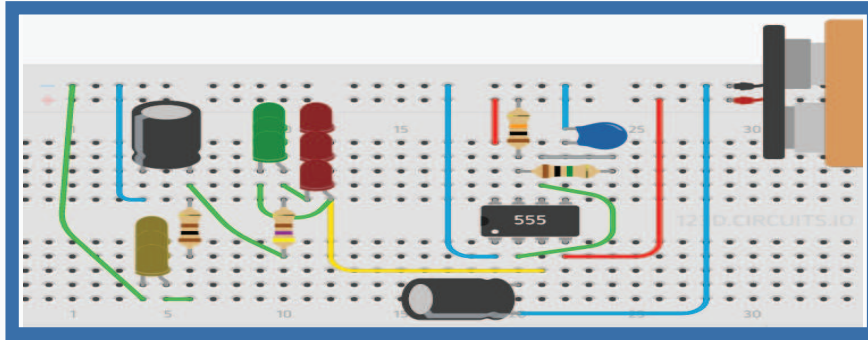
مخطط تركيب دائرة المشروع باستخدام موقع 123dapp
