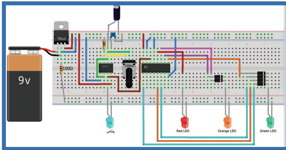
دائرة الإشارة الضوئية
