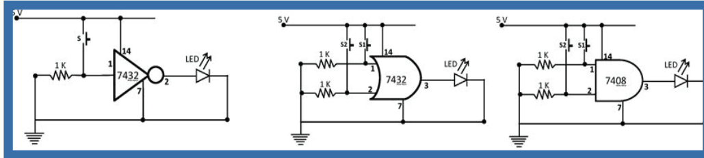
دارات مقترحة للبوابات المنطقية الأساسية
