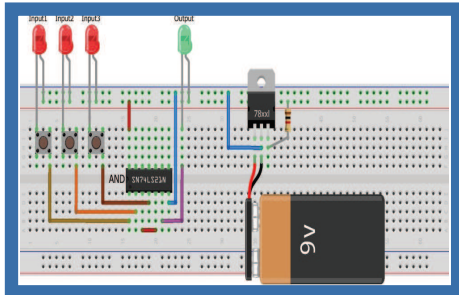
دائرة توصيل بوابات بأكثر من مدخلين
