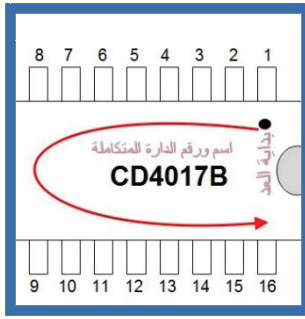
أرجل الدارة المتكاملة
