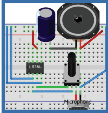
مخطط توصيل دائرة الصوت
