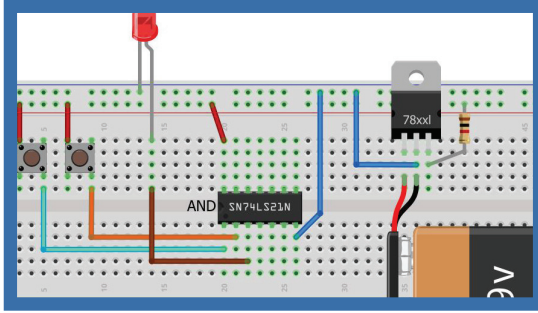
دائرة البوابة AND
