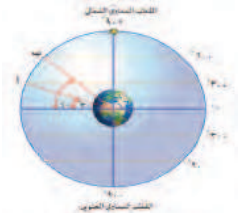
الشكل (١١-ب): الميل الاستوائي
