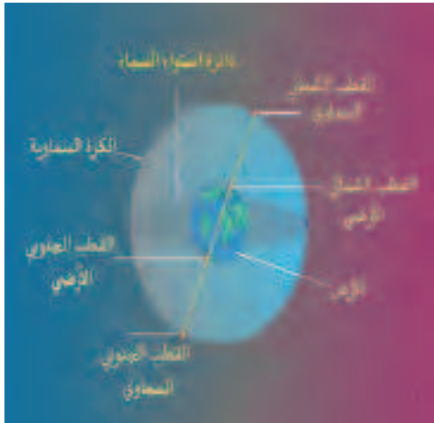
الشكل (٥): دائرة استواء السماء والقطين السماويين
