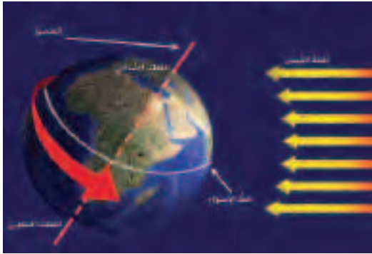
الشكل (١٤) : دوران الأرض حول نفسها
