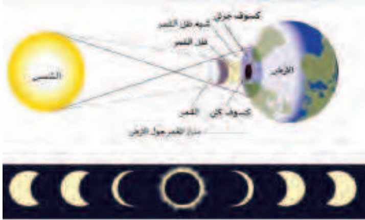
الشكل (٢٢): خسوف الشمس
