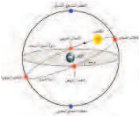
الشكل (١٠): دائرة البروج
