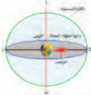
الشكل (٦): سمت الرأس والنظير
