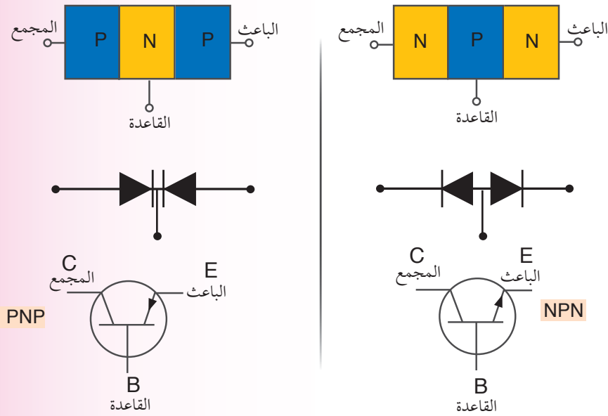
تمثيل الترانزستور
