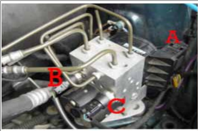
شكل (١٥): وحدة التحكم الهيدروليكي لنظامي ABS و TCS
