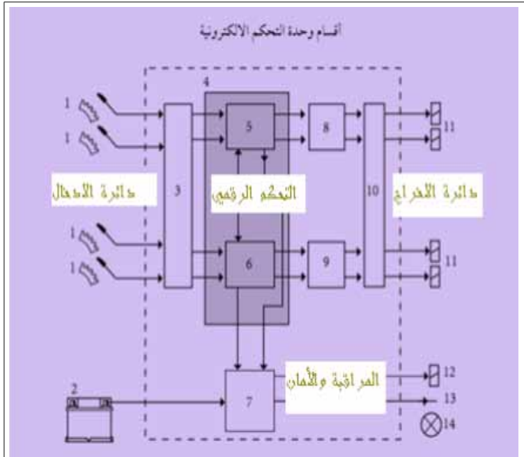
شكل (٥): أقسام وحدة التحكم الإلكترونية
