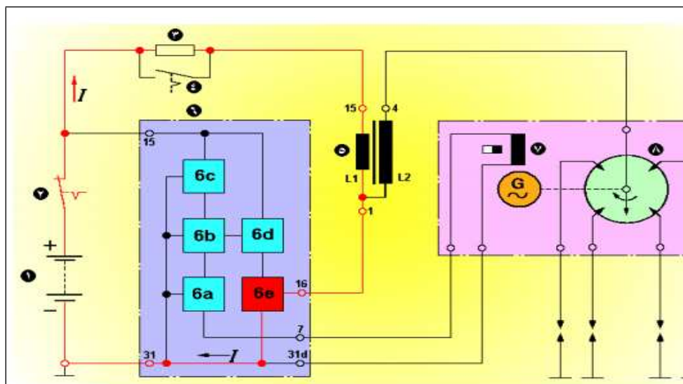
الشكل (١) الأجزاء الرئيسية لنظام الإشعال ذي مولد النبضة الحثي (الملف اللاقط)
