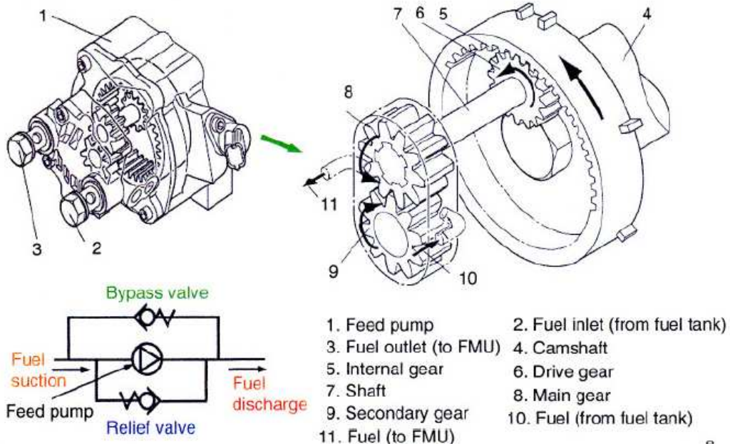
شكل (١٨): مضخة التغذية
