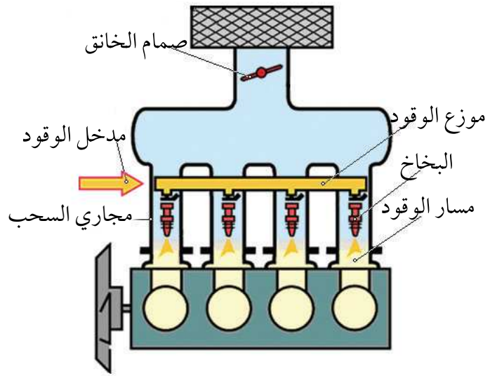
شكل (١٤) نظام الحقن الالكتروني متعدد النقاط
