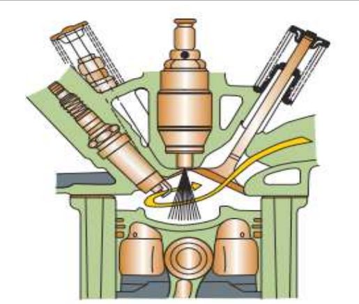
الشكل (١٦) حقن الوقود مباشرة في غرفة الاحتراق
