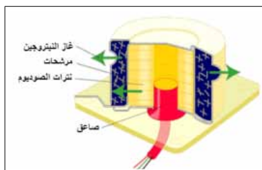
شكل (٤٣): مكونات مولد الغاز
