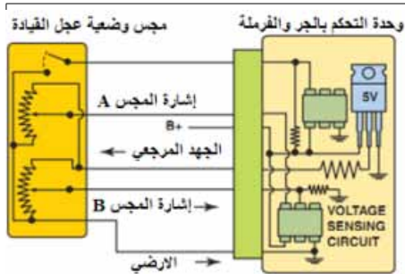
شكل (٢٤): توصيل مجس وضعية عجلة القيادة مع وحدة التحكم
