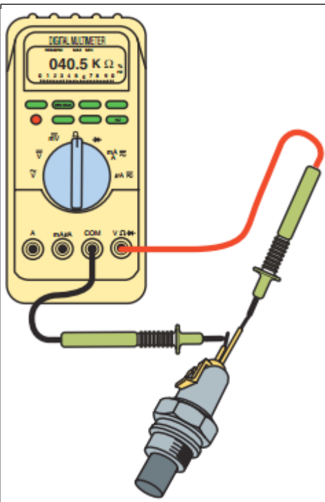
الشكل (٤٧) تأثير الحرارة على مقاومة المجس
