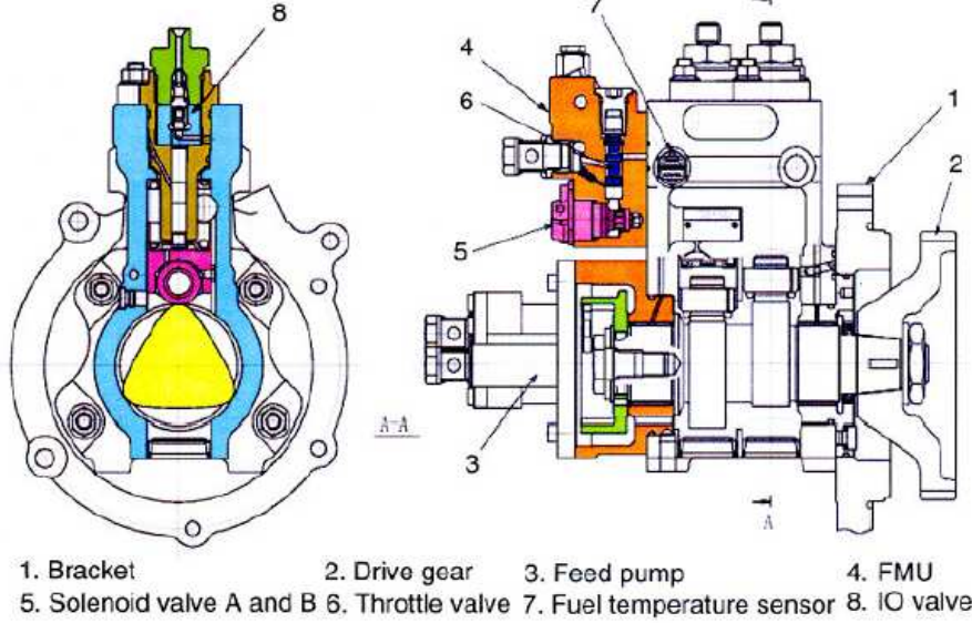
شكل (١٧): مقطع مضخة الديزل
