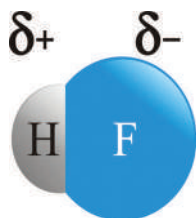
الشكل (4): تمثيل الرابطة القطبية في جزيء H-F
