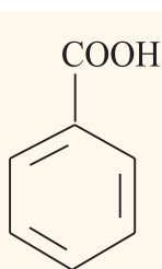
حمض البنزويك
