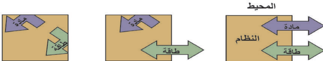
الشكل (4): تبادل المادة والطاقة في الأنظمة الحرارية
