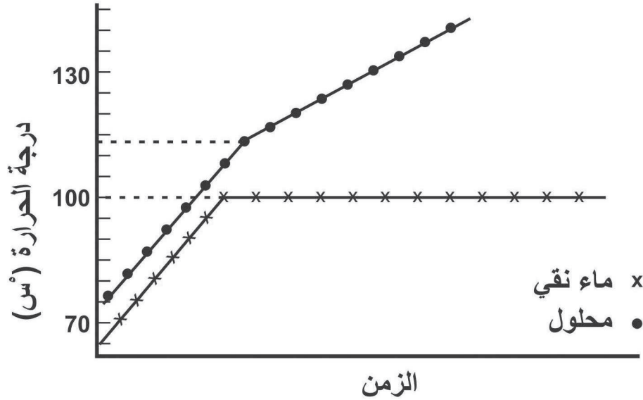
الشكل (4): منحنى درجة الغليان للماء النقي، ومحلول السكر في الماء
