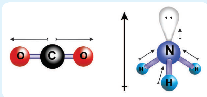
جزيء \text{CO}_2
