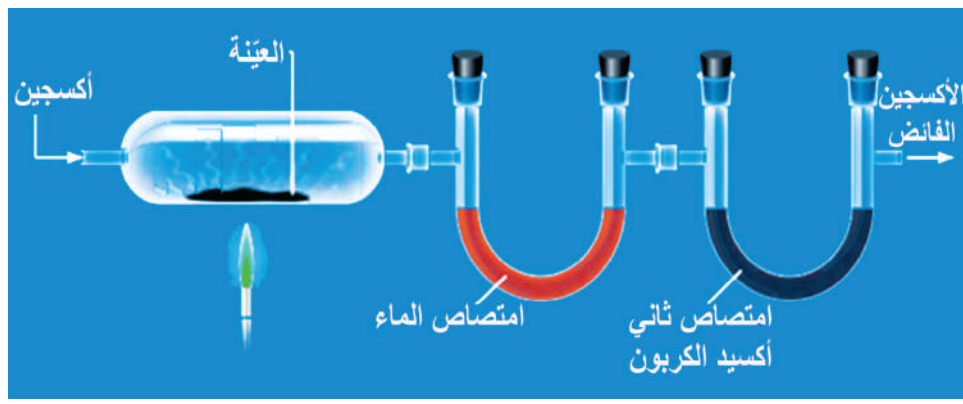
الشكل (1): عملية حرق عينة من مركب عضوي؛ لإيجاد صيغته الأولية
