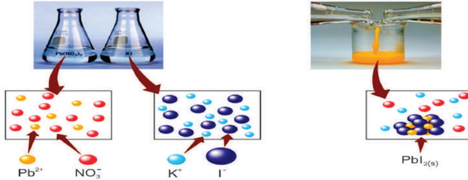
الشكل (6): توضيح تمثيلي لتفاعل محلولي نترات الرصاص (II)، ويوديد البوتاسيوم
