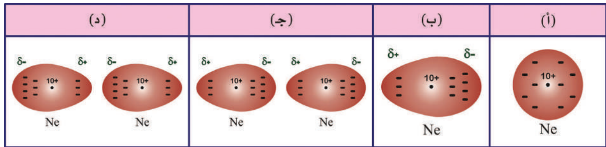
الشكل (8): تمثيل قوى لندن بين ذرتي نيون
