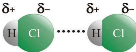
الشكل (5): تمثيل قوى التجاذب بين الجزيئات القطبية لجزيئات HCl
