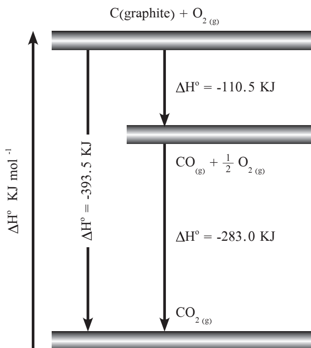
الشكل (7): حساب المحتوى الحراري لتكوين CO_2 بشكل غير مباشر
