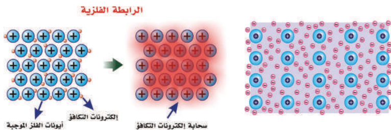
الشكل (2): تمثيل الرابطة الفلزية
