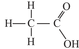
حمض الأسيتيك (يوجد في الخل)
