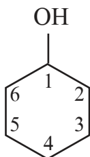
سايكلو هكسانول
