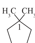
1،1-ثنائي ميثيل سايكلو بنتان
