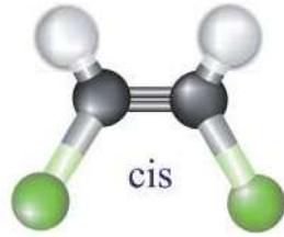
م-1،2-ثنائي كلورو إيثين
