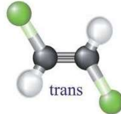
ض-1،2-ثنائي كلورو إيثين
