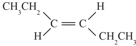
ض-3-هكسين
