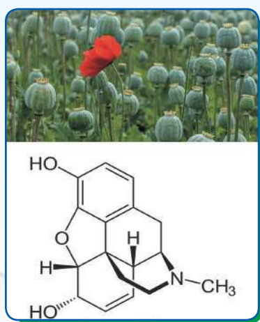
Morphine مورفين
