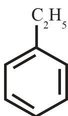
إيثيل بنزين
