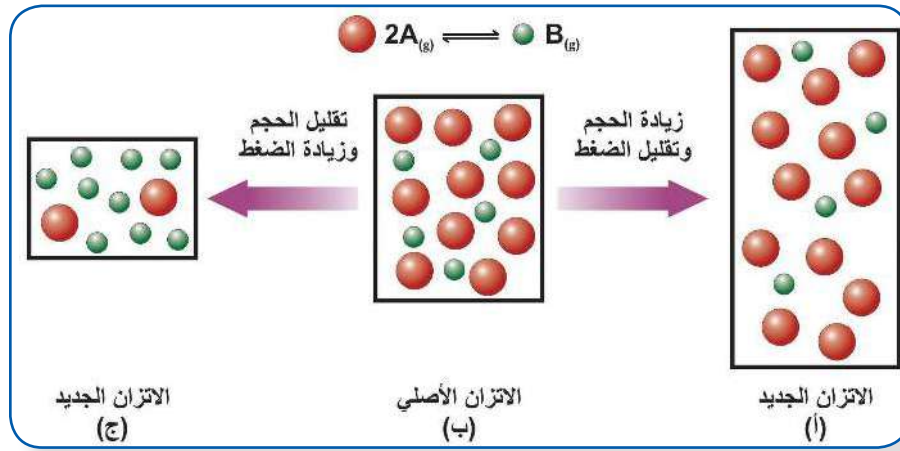
الشكل (2): أثر تغيُّر الضغط الخارجي على حالة الاتزان
