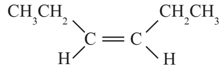
م-3-هكسين
