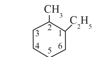
1-إيثيل-2-ميثيل سايكلو هكسان
