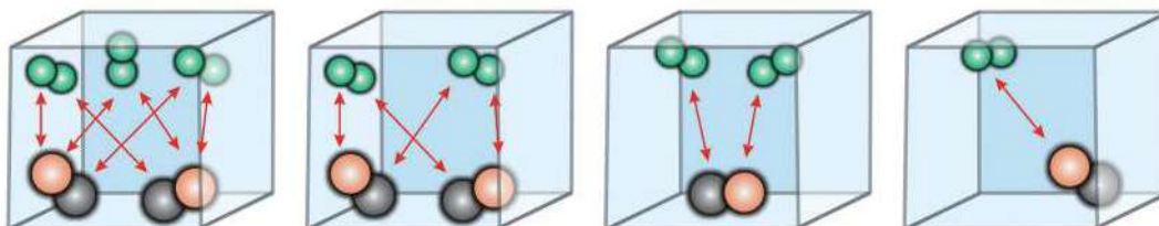
الشكل (1): تمثيل للتصادمات المحتملة بين جزيئات \text{NO} و \text{Cl}_2
