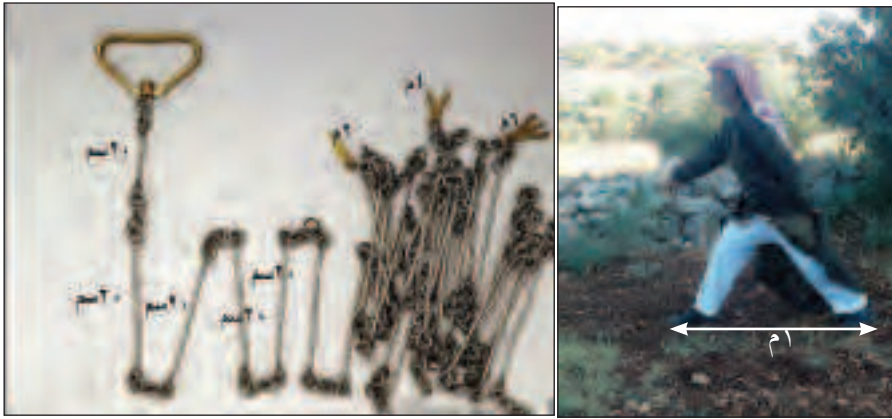
صورة (٢): الجنزير
