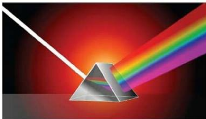
الشكل (1-3) خطوط الطيف المتصل
