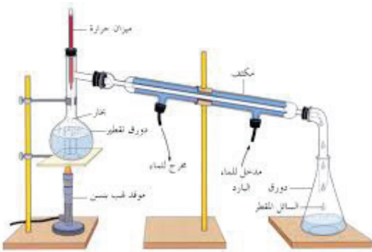
الشكل (١١): جهاز التقطير البسيط
