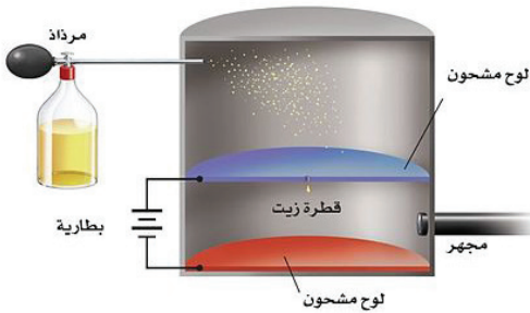
الشكل (2): تجربة ميليكان
