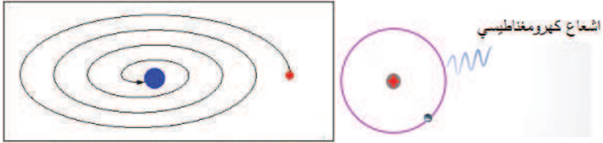
الشكل (11): المسار المتوقع للإلكترون أثناء دورانه حول النواة
