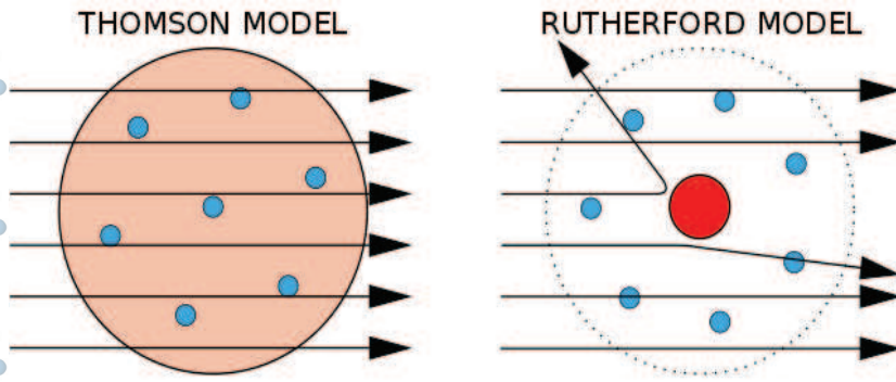
الشكل (10): فروق بين نموذج رذرفورد ونموذج ثومسون.
