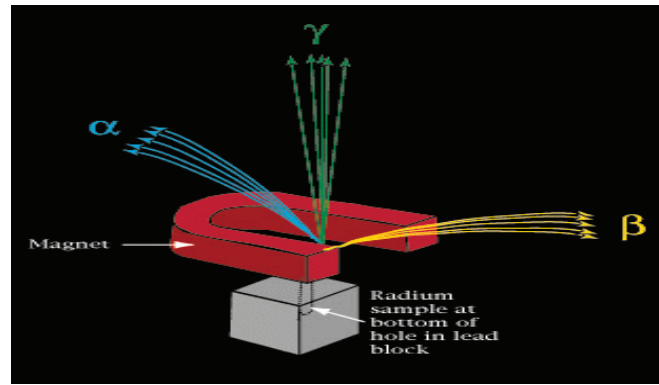
الشكل (٤): تفاوت سلوك الأشعة الصادرة عن العناصر المشعة عند تعرّضها للمجال المغناطيسي
