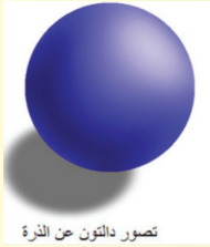
تصور دالتون عن الذرة
