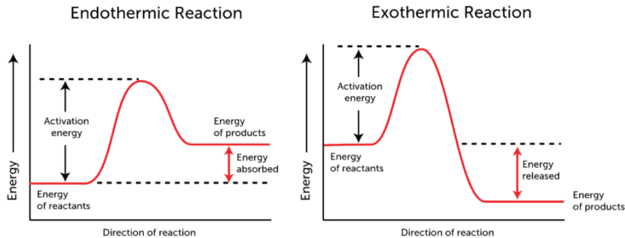
الشكل (١٣): الفرق بين منحنى التفاعل الطارد للطاقة والماص لها
