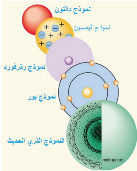
الشكل (12): تطور مفهوم بنية الذرة
