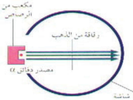
الشكل (7): توقعات رذرفورد لسلوك أشعة ألفا خلال صفائح الذهب، اعتماداً على نموذج ثومسون
