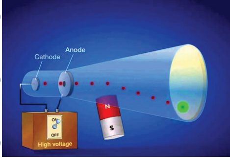
الشكل (1): تجربة ثومسون
