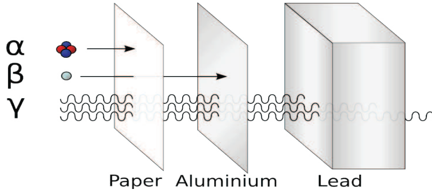
الشكل (5): تفاوت الأشعة الصادرة عن العناصر المشعة في اختراق بعض الأجسام
