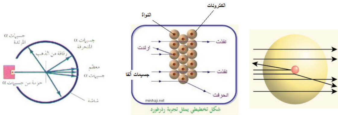
الشكل (8): نتائج تجربة رذرفورد
