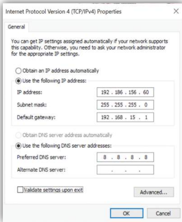
7. يمكن اختيار الاعداد اليدوي لتعيين عنوان ثابت (Use The Following IP Address)
