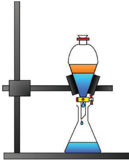
قُمع الفصل
