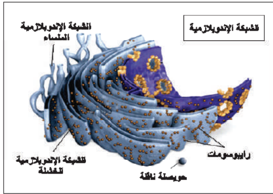
الشكل (3) الشبكة الاندوبلازمية
