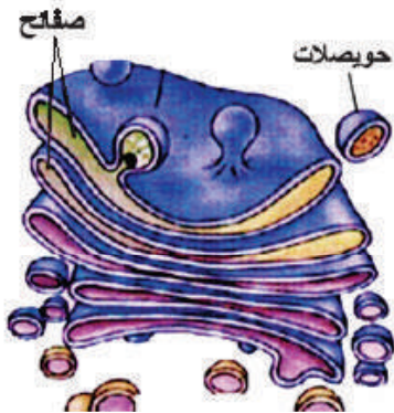
الشكل (4) جهاز غولجي
