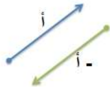
متجهان متعاكسان
