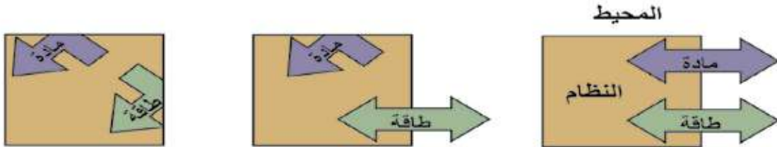
الشكل (6): تبادل المادة والطاقة في الأنظمة الحرارية
