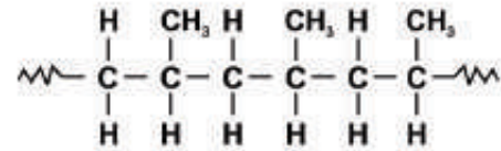
مقطع من بوليمر البولي البروبيلين
