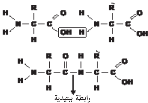
الشكل (9-3): ارتباط حمضين أمينيين
