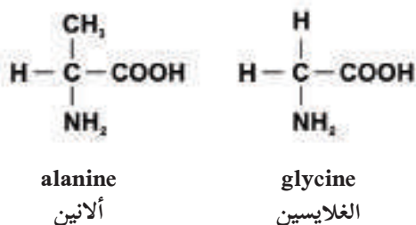
الشكل (9-3): ارتباط حمضين أمينيين
