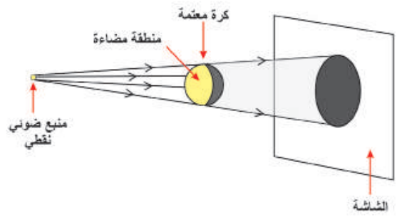
شكل (أ): منطقة الظل عندما يكون مصدر (منبع) الضوء نقطياً
