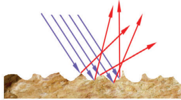
انعكاس غير منتظم عن السطوح الخشنة
