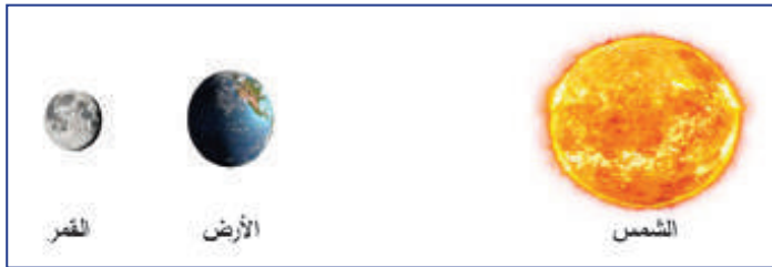
الشكل (ب): صورة تقريبية تحاكي خسوف القمر
