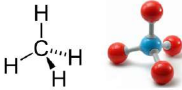
الشكل (1): الصيغة البنائية للميثان
