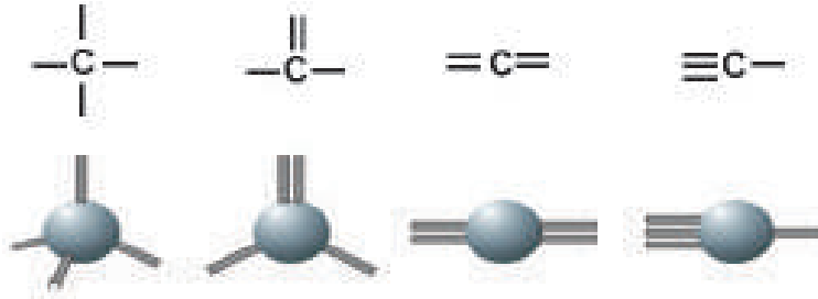
الشكل (3): أنواع الروابط التي يكونها عنصر الكربون
