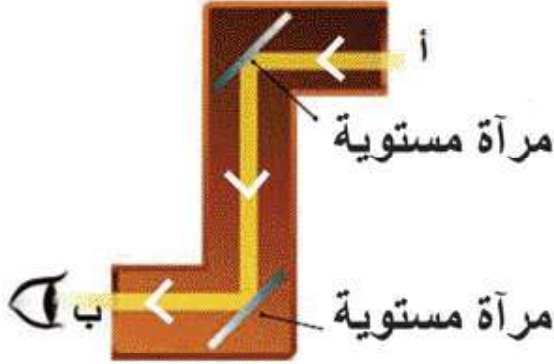
شكل ( ١ ) أنموذج لبريسكوب بسيط
