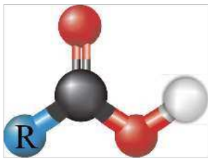
الصيغة العامة للحموض الكربوكسيلية
