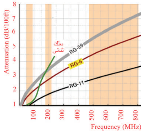
شكل (2): منحنيات الخواص الترددية لعدة أنواع من خطوط النقل
