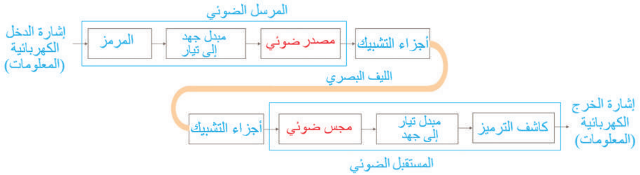
شكل (8): المخطط الصندوقي لنظام اتصالات الألياف البصرية
