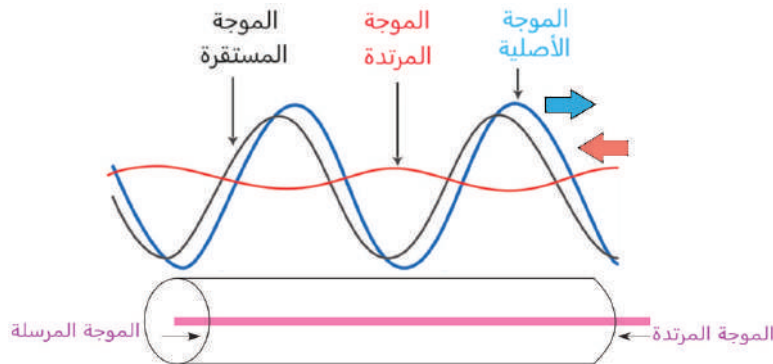
شكل (6): الأمواج الموقوفة (المستقرة) على خط النقل كمحصلة لتداخل الأمواج المرسلة والأمواج المرتدة
