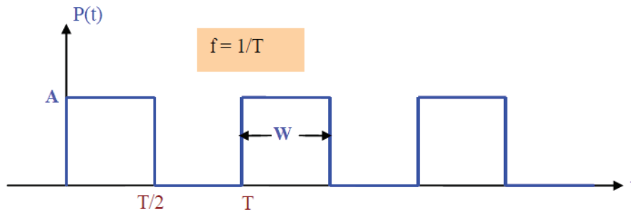
شكل (2) النبضات المربعة أحادية القطبية
