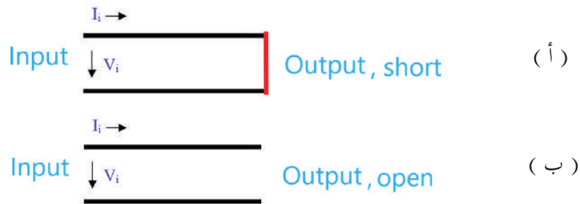
شكل (2): أ- نهاية خط النقل مقصورة (Short) عند قياس R و L ب- نهاية خط النقل مفتوحة (Open) عند قياس C
