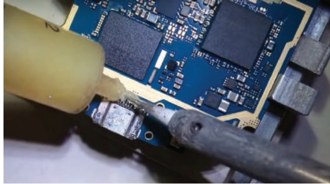
شكل (7): وضع الفلنكس للمساعدة في فك القاعدة
