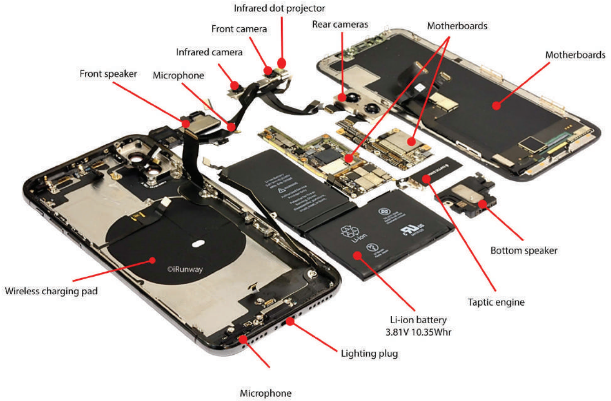
شكل (15): المكونات الرئيسية لأحد أجهزة آيفون (iPhone)
