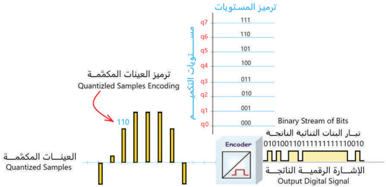
شكل (8): مبدأ عمل مرحلة الترميز (مع وجود محول توازي-توالي)
