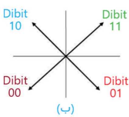
شكل (5): الحالات المميزة لنظام التضمين QPSK، (أ): الأشكال الموجية (ب): مخطط المتجهات
