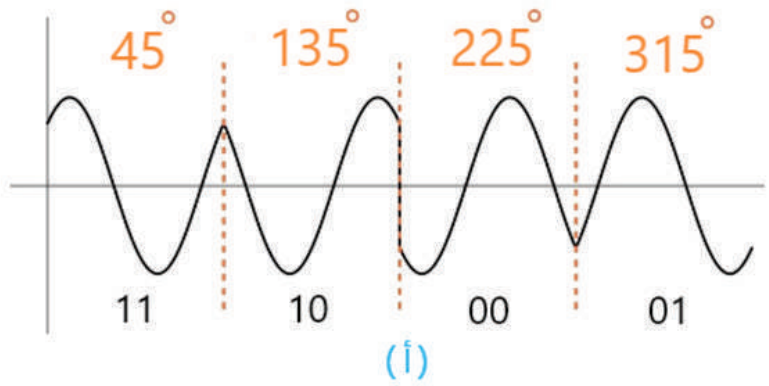
شكل (5): الحالات المميزة لنظام التضمين QPSK، (أ): الأشكال الموجية (ب): مخطط المتجهات
