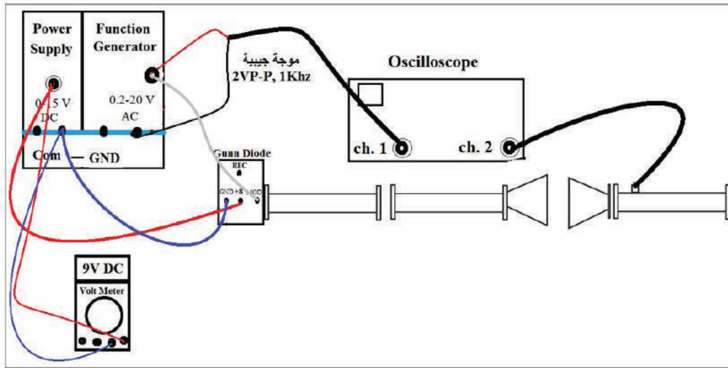
شكل (2): إرسال ميكرويف مضمّن باستخدام مذبذب Gunn
