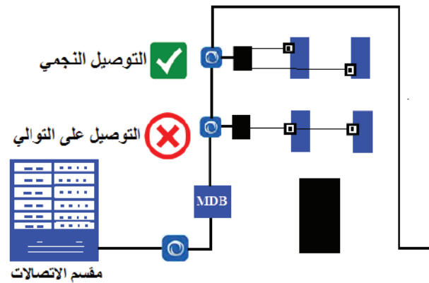
شكل (7): توصيل نجمي وتوصيل توالي
