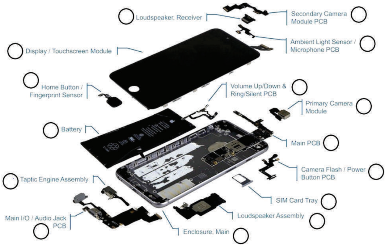
شكل (13): المكونات الأساسية لأحد الهواتف الذكية (Plus 6S iPhone)
