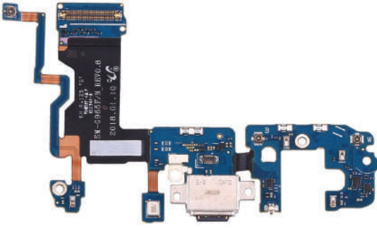
شكل (8): فلات شحن لجهاز (Samsung Galaxy S9)
