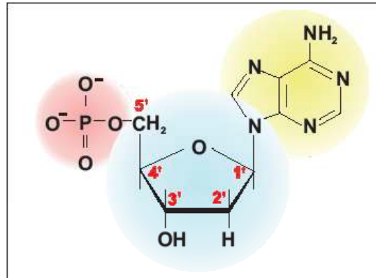
(أ) نيوكليوتيد ل DNA
