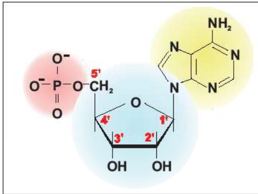
(ب) نيوكليوتيد ل RNA
