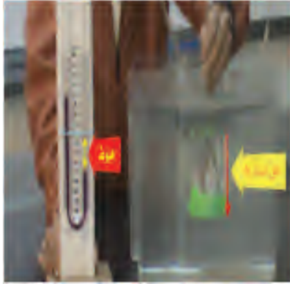
الشكل (٣-٥): العلاقة بين ضغط السائل وعمقه
