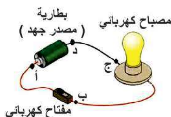
الشكل (٤): دائرة كهربائية بسيطة
