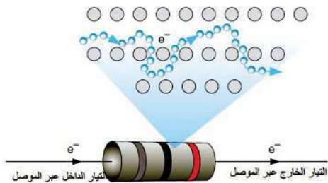
الشكل (١) حركة الإلكترونات الحرة في الموصل
