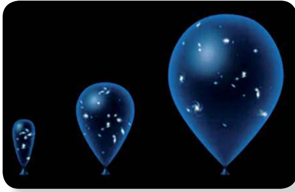
الشكل (٣) توسع الكون
